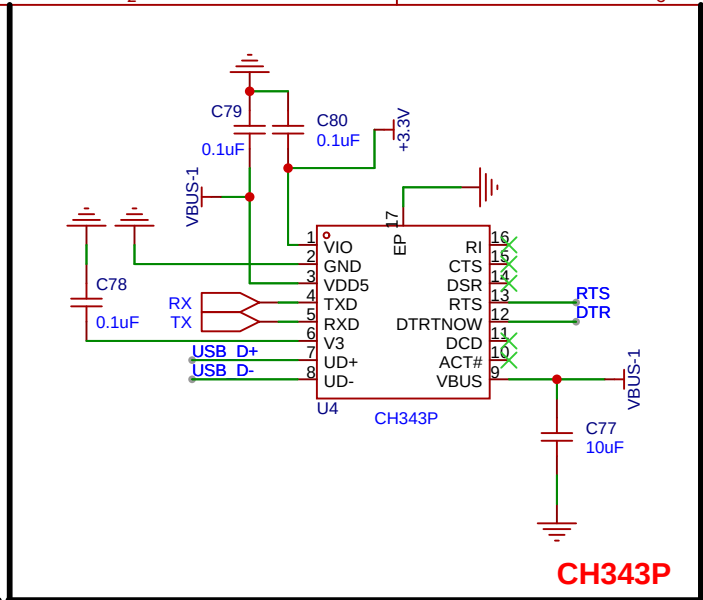
UART
